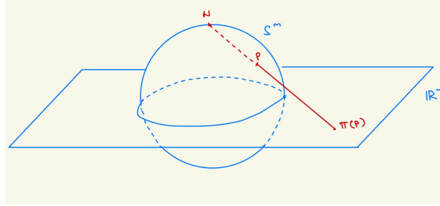
La proiezione stereografica
