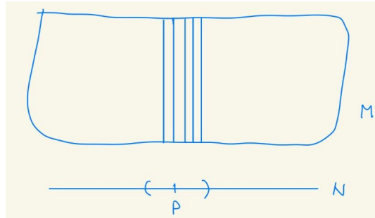
Esempio di fibrato
